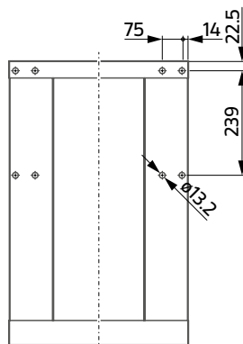
Schubladenschrank (sämtliche Breiten) Schuifladenkast (alle breedtes) Armadio a cassetti (tutte le dimensioni) Armario de cajones (todas las dimensiones) Drawer cabinet (all width)
