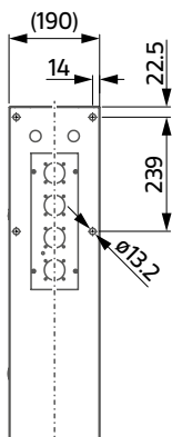
Aggregatschrank Aggregaatkast Armadio per allacciamenti Armario de grupos Power unit cabinet
